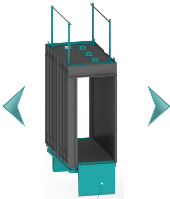
کابین دو درب تونلی
